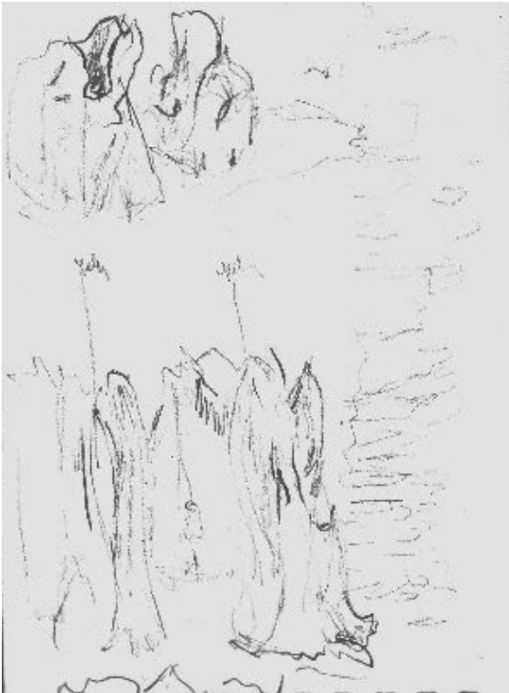
16a PINNACLES, NAMBUNG NAT. PK., W.A.
